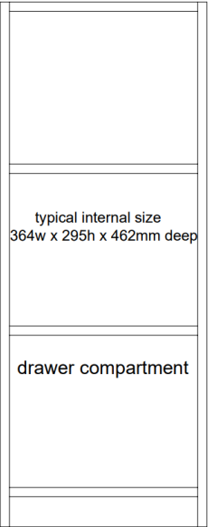
2 DOOR / 1 DRAWER
